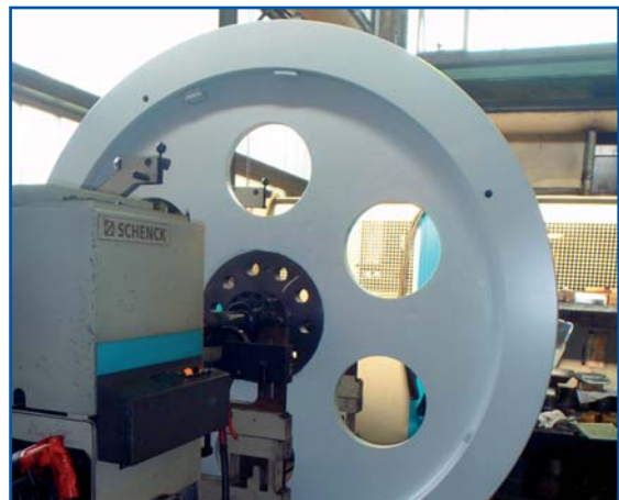
Dynamisches Auswuchten in zwei Ebenen nach DIN 1940
