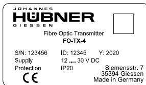
Abb. 4-1: Typenschild (Beispiel)
